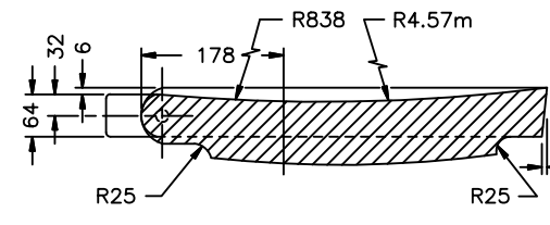
SECTION D-D
