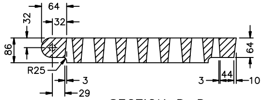
SECTION D-D
