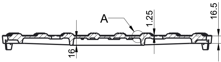
SECTION A-A
